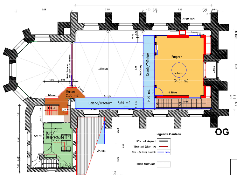
Bild: Der Plan für das Obergeschoss der Alten Kirche.
